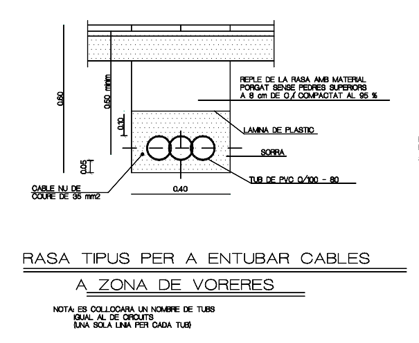
RASA TIPUS PER A ENTUBAR CABLES A ZONA DE VOREIRES
