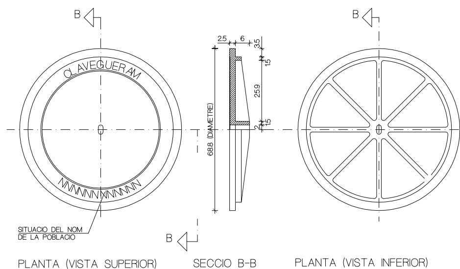
PLANTA (VISTA SUPERIOR)
