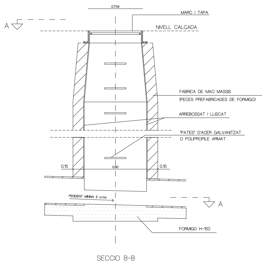
SECCIO B-B
