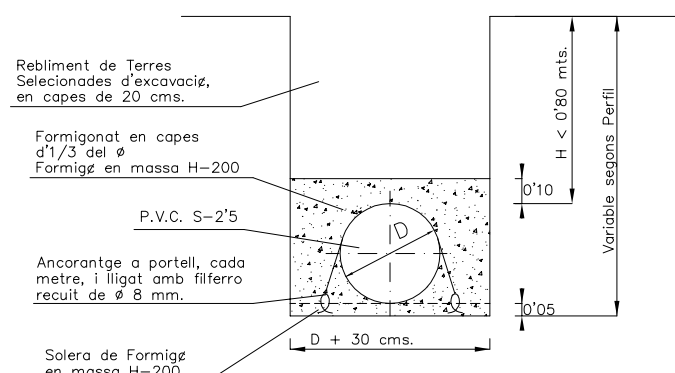
CONDUCCIONS DE CLAVEGUERAM
