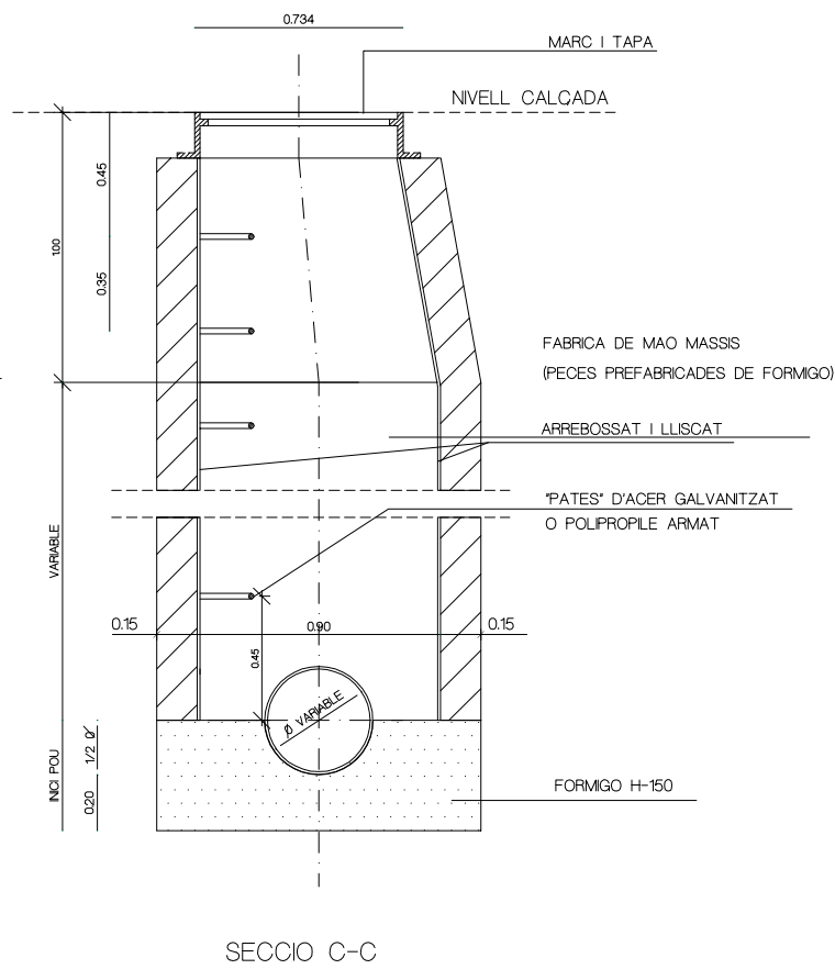
SECCIO C-C
