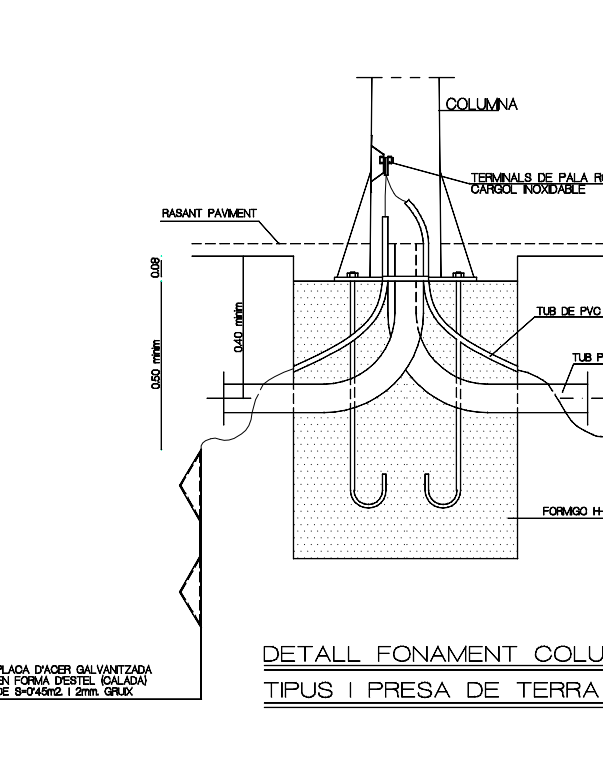
DETALL FONAMENT COLUMNA TIPUS I PRESA DE TERRA
